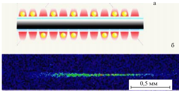
Рис. 7. (а) Нановолновод с локализованными вокруг него атомами. (б) Изображение облака атомов Cs, локализованных вокруг нановолновода, полученное с помощью ПЗС-камеры (ПЗС — прибор с зарядовой связью) [29].
