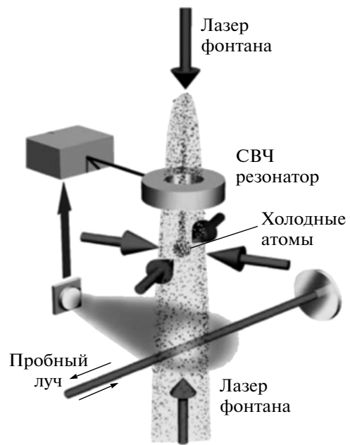
Рис. 3. Схема атомного фонтана
