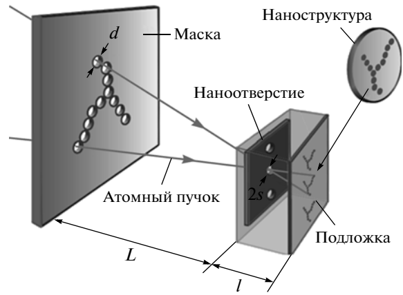
Рис. 6. Схема атомной камеры-обскуры Атомы, прошедшие через отверстия в маске, формируют, по аналогии со световой оптикой, “светящийся объект” заданной геометрии. С помощью нанотверстия на подложке создается атомная наноструктура – уменьшенная копия маски
