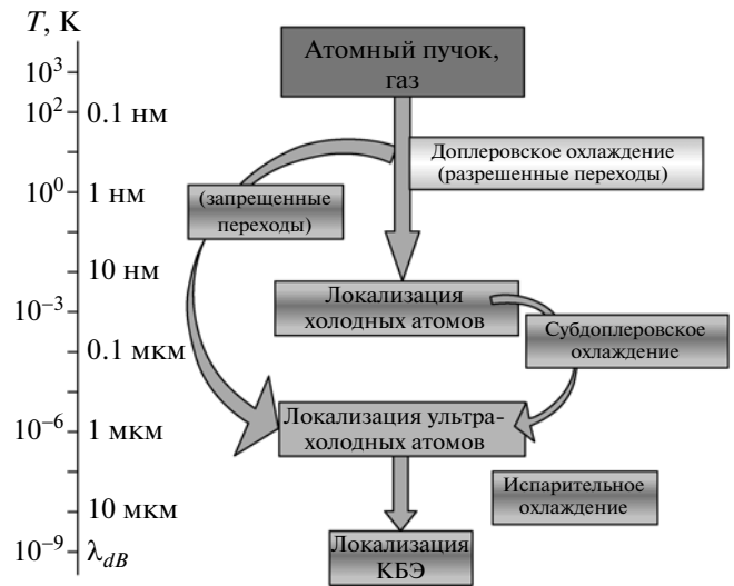
Рис. 1. Основные физические механизмы лазерного охлаждения нейтральных атомов
