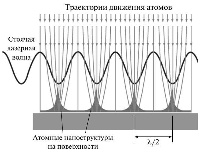
Рис. 4. Атомная линза, образованная стоячей световой волной
