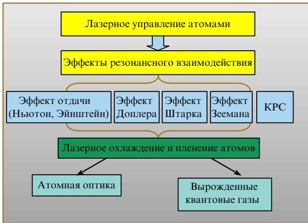
Рис. 1. Схема, иллюстрирующая роль эффектов атомной физики (эффекта отдачи, эффектов Доплера, Штарка, Зеемана и эффекта комбинационного рассеяния света) в развитии методов лазерного охлаждения и плениения атомов и атомной оптики.
